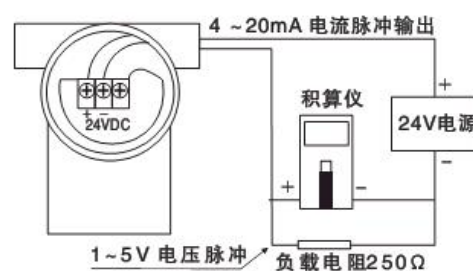
脉冲输出为二线制
