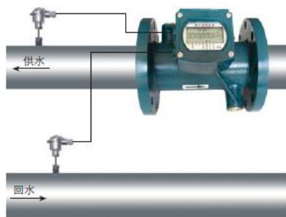
机械尺寸图详见<12页>超声波工业水表
