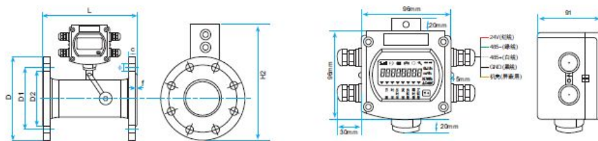
大口径水表机械尺寸 (单位: mm)
