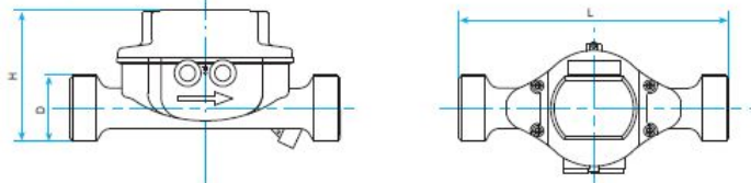
小口径水表机械尺寸 (材质: 精铸不锈钢316L)
