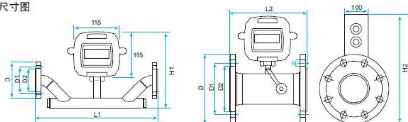
■ 法兰管段式尺寸图
