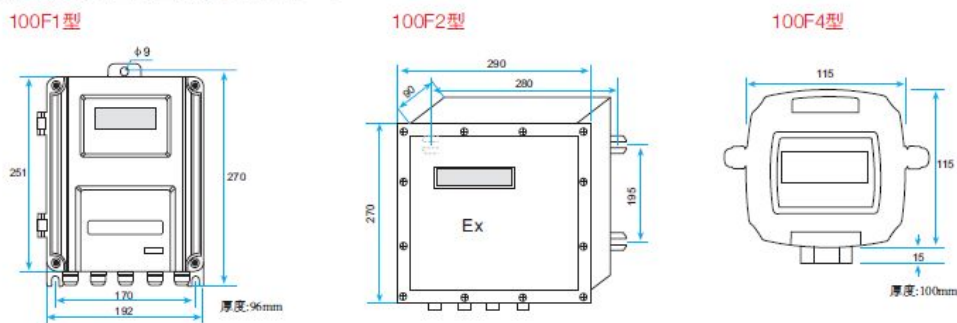
■ 主机外形尺寸图及主板接线图(单位:mm)
